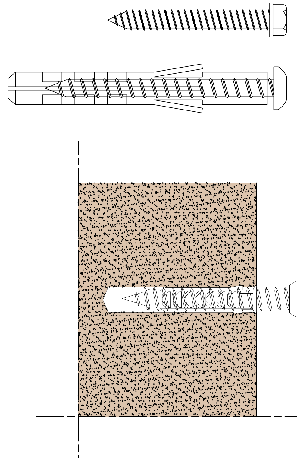
ΤΟΠΟΘΕΤΗΣΗ ΒΙΔΑΣ
