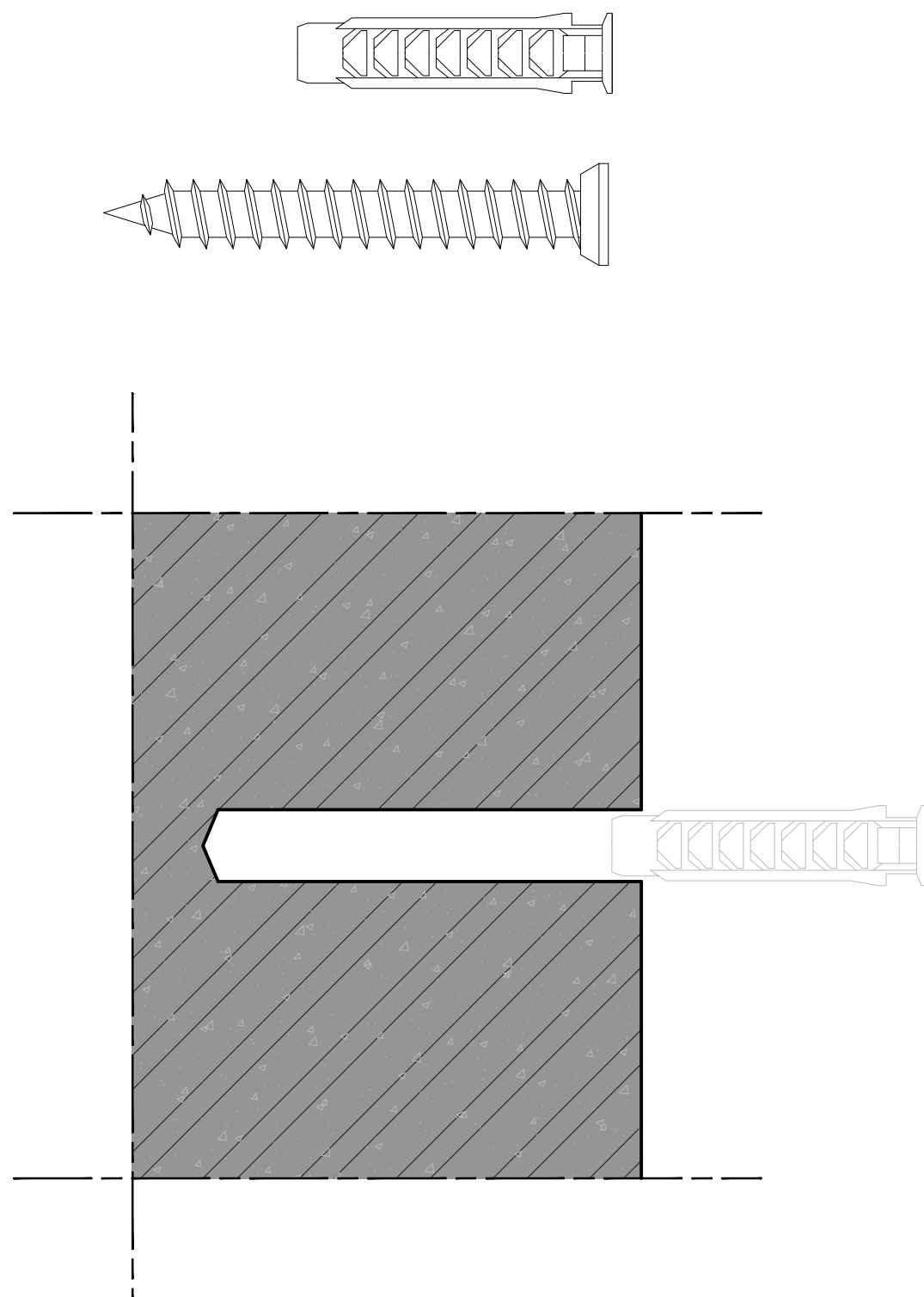
ΤΟΠΟΘΕΤΗΣΗ ΟΥΠΑΤ
